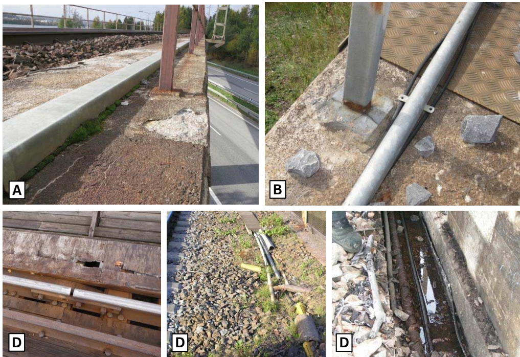
Kuva 18. Ylärivissä vasemmalla johdot ovat asiallisesti suojakourun sisällä, mutta oikeanpuoleisella sillalla kunnossapitäjän on siistittävä johdot suojakourun alle takaisin ja laitettava kouru kunnolla kiinni.
