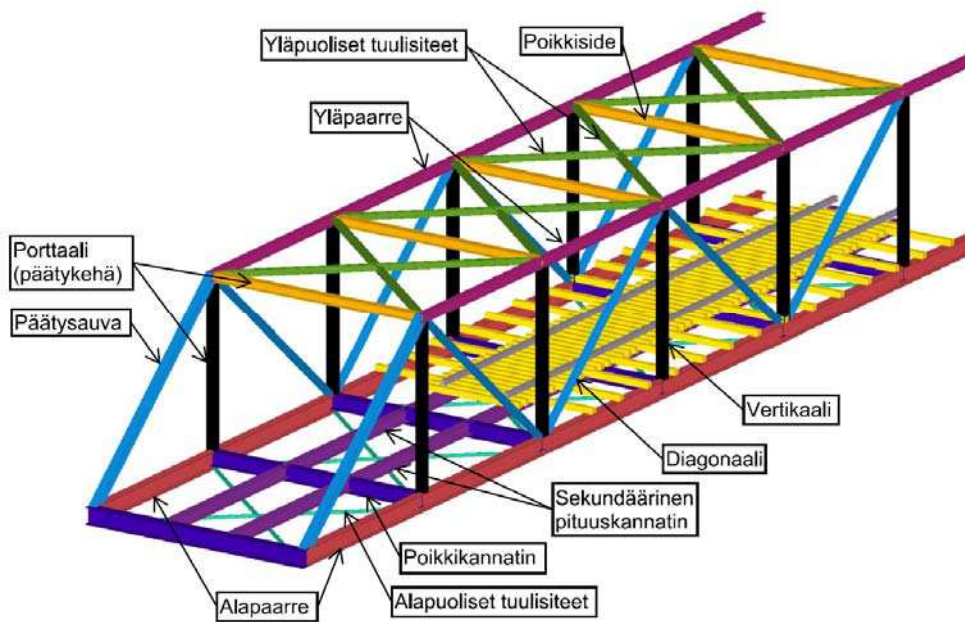
Kuva 7. Teräsristikkosiltaan liittyvät rakenteet
